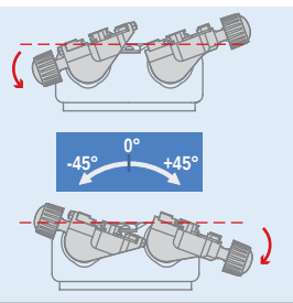
Наклонный зажим (0° +/- 45°) с четырьмя местами ключевого позиционирования
